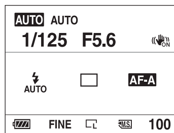
Interfața standard
