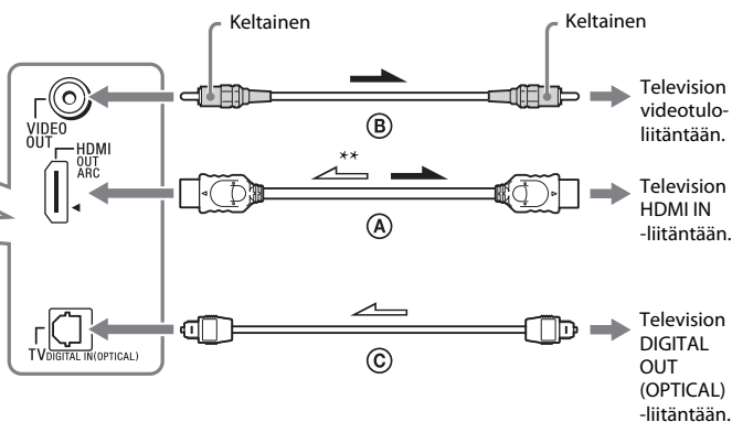
Päälaitteen takapaneeli
